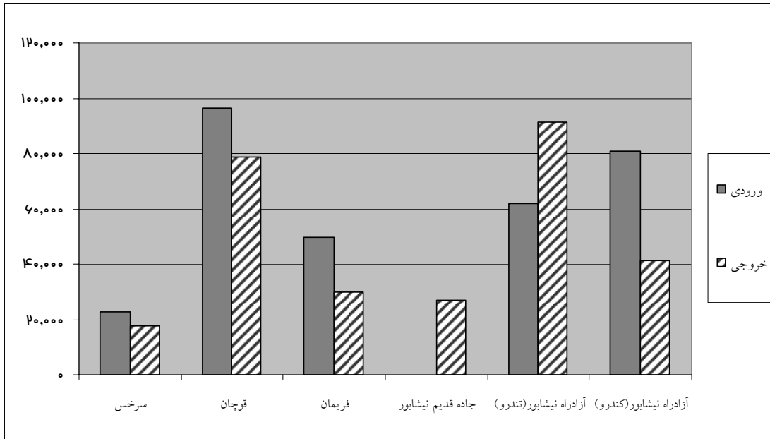
نمودار شماره (۱): حجم ترافیک ورودی به و خروجی از مشهد در محورهای شش گانه ۲۲ تا ۲۸ تیرماه ۱۳۸۶
